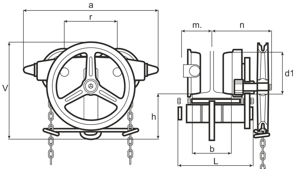
Dane techniczne i wymiary gabarytowe serii HRW-EX
