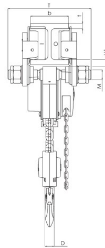
5000 kg; 2-ciężnowy
