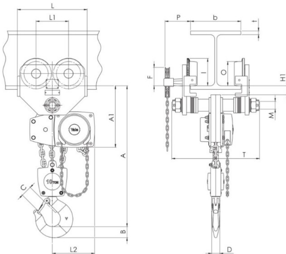
10 000 kg; 3-ciężnowy
