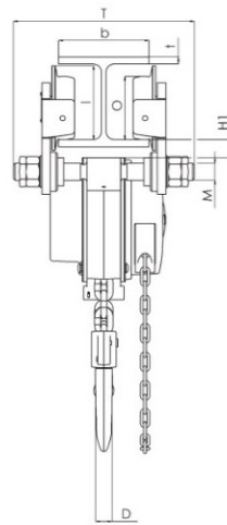
500 - 3000 kg; 1-ciężnowy
